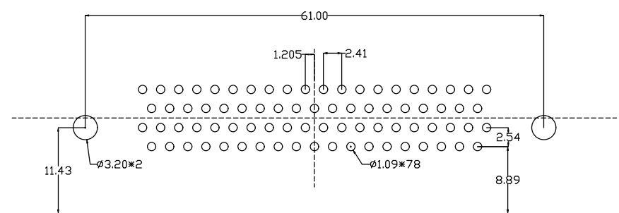
P.C.B LAYOUT
