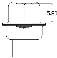
B=前铆5.8实心螺母
